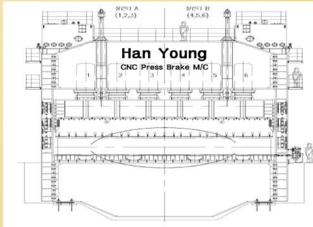
벤딩시 처짐현상 참조도면
